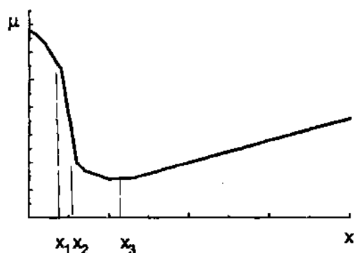
Рис. 2. Схематичний хід залежності коефіцієнта тертя \mu від приведеної швидкості x=\eta v/\rho ( \eta – в'язкість, \rho – густина) [1]
