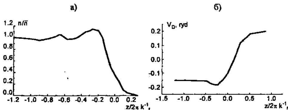
Рис. 1. Розподіл а) відношення концентрації n/\bar{n} носіїв та б) потенціалу дипольного шару V_D у напрямку нормалі до поверхні (за даними [7,8])
